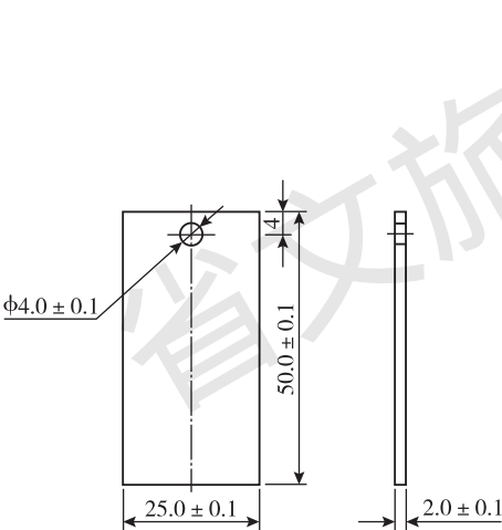
图 B.1 I 型试片
