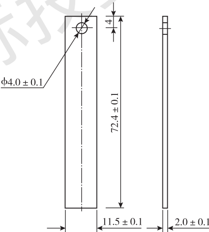
图 B.2 II 型试片
